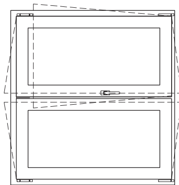
FINESTRA 2 ANTE - A/R D1210031 - D1210032
