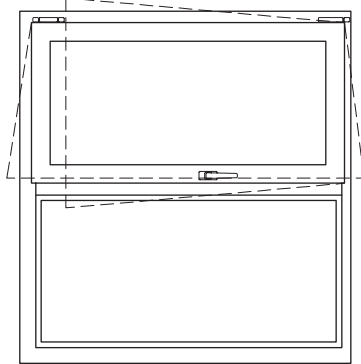
FINESTRA 1 ANTA - A/R + FISSO LAT. D0062513 - D0062515
