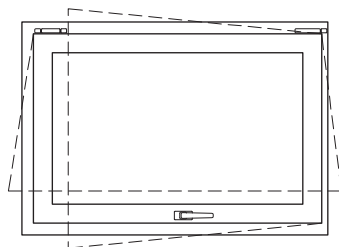
FINESTRA 1 ANTA - A/R D0062513 - D0062515
