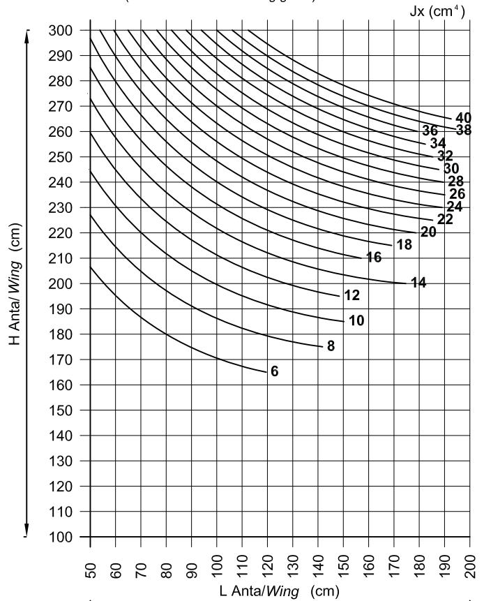
CARICO DEL VENTO/ WIND LOAD : q= 50 Kg/m 2 f max H/300 (Vetro isolante / insulating glass)
