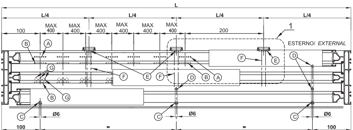
3 ANTE / WINGS
