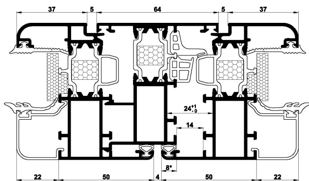
nodo centrale
