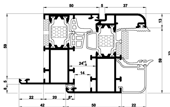
nodo laterale
