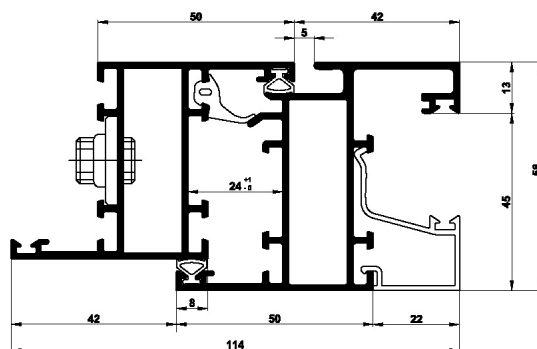
nodo laterale
