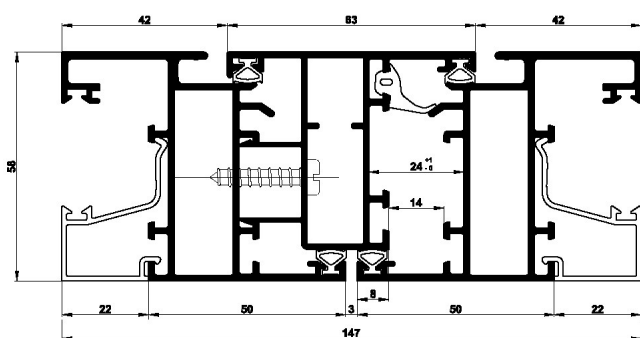
nodo centrale
